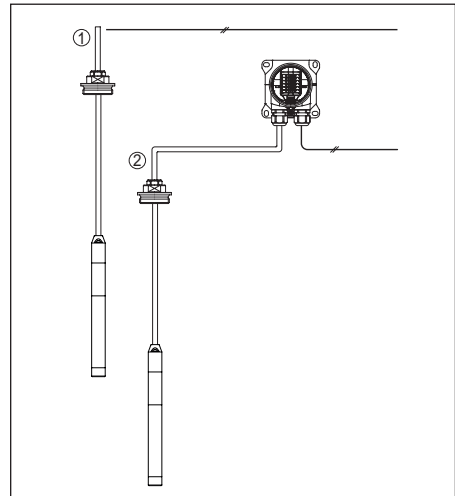
Abb. 24: Raccordement du VEGAWELL S 51 à l'alimentation
