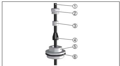
Abb. 23: Structure du bouchon fileté pour câble porteur
