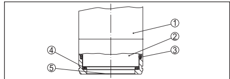
Abb. 20: Montage arasant de la cellule de mesure CERTEC® avec joint double
