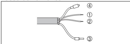
Abb. 25: Occupation des conducteurs câble porteur
