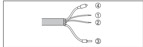
Abb. 34: Ocupación de conductores del cable portador
